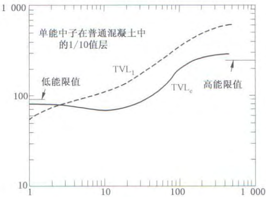
图 C.3 中子在混凝土中的 1/10 值层
